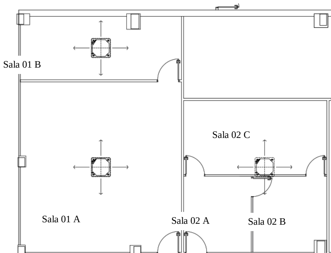
Planta baixa da localização dos equipamentos de Ar Condicionado
