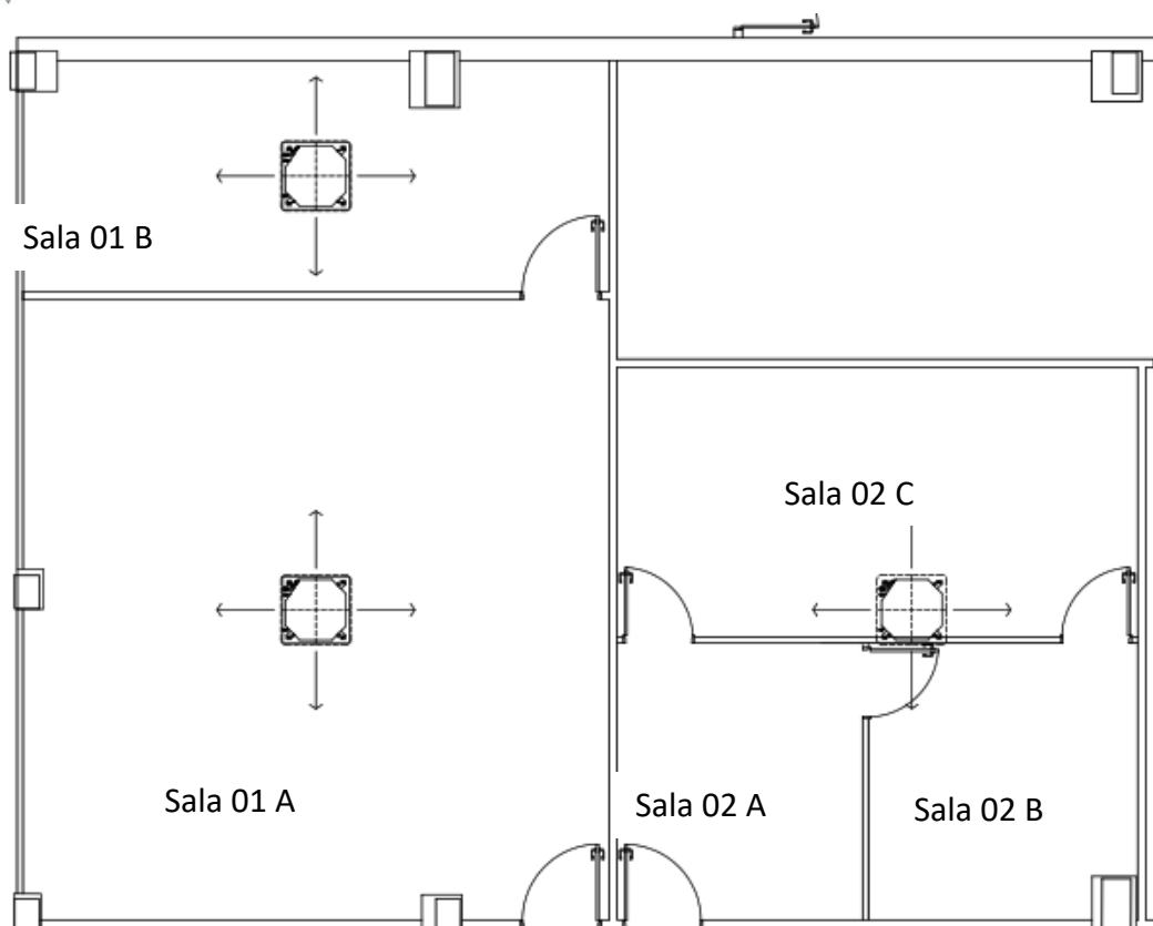
Planta baixa da localização dos equipamentos de Ar Condicionado
