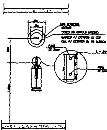
VISTA FRONTAL DET. DE EXTINTOR FIXADO NA ALVENARIA OU NO PILAR SEM ESCALA
