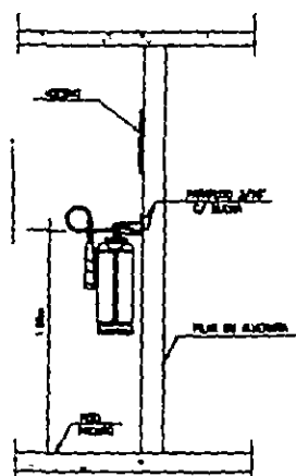
VISTA LATERAL DET. DE EXTINTOR FIXADO NA ALVENARIA OU NO PILAR SEM ESCALA
